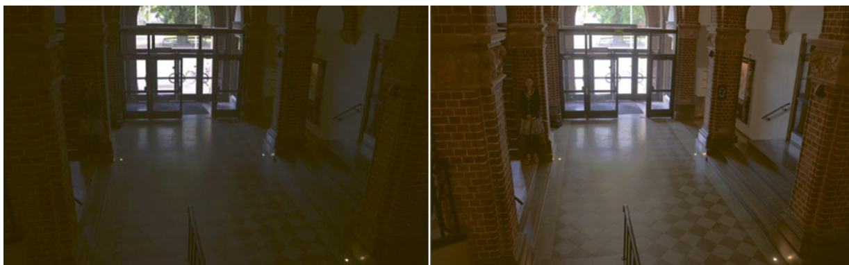
Figure 4. Von hinten beleuchteter Innenraum, erfasst von Kameras mit unterschiedlichem dB-Wert. Wider Erwarten stammt das rechte Bild von einer Kamera, deren angegebener dB-Wert geringer war als bei der linken Kamera.
